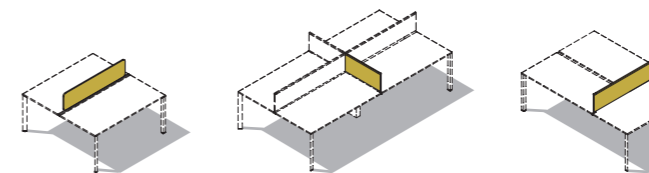
W 100 / 140 / 160 / 180 D 1,8 - H 36 W 80 D 1,8 - H 32,9 / 37,1 W 160 D 1,8 - H 31,1 / 32,9 / 35,3 / 37,1
