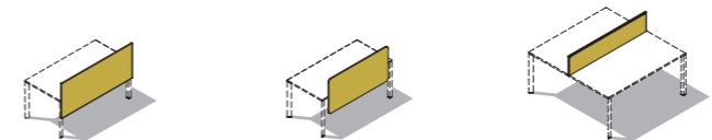
Screen W 120 / 140 / 160 / 180 / 200 D 1,8 - H 68,5 / 70,3 W 96 / 116 / 136 / 156 / 176 D 1,8 - H 69 W 120 / 140 / 160 / 180 / 200 D 1,8 - H 31,1 / 32,9 / 35,3 / 37,1
